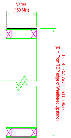
Section A-A
